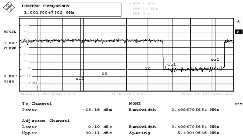
Fig. 8 FSP ACP Display
