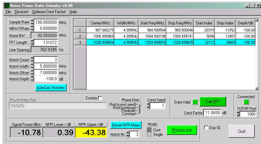
Fig. 2 Main Menu
